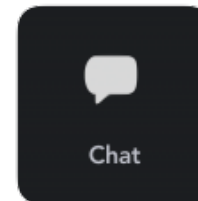
Zoom Chat
